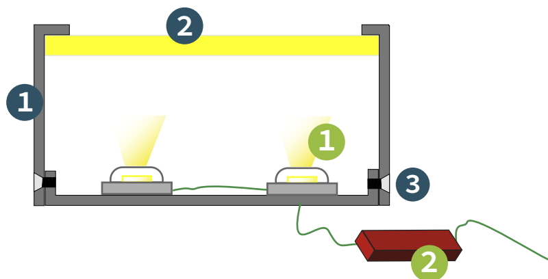
SCHÉMA
